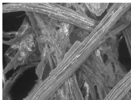
茶葉・葉脈繊維の電子顕微鏡写真（200倍）
